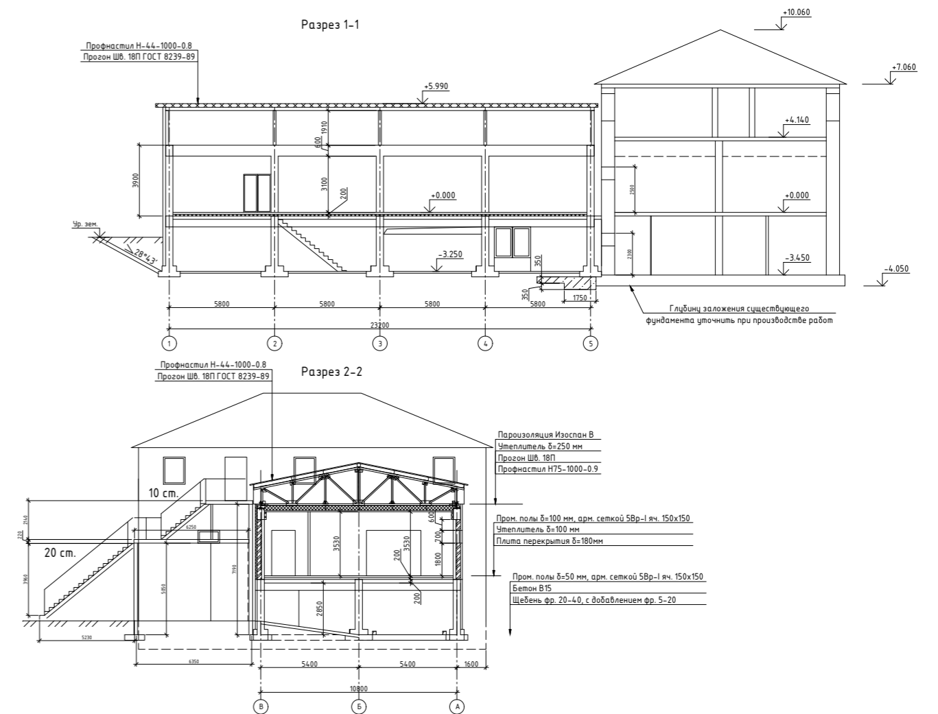
Разрезы 1-1, 2-2
