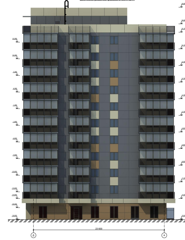
Фасад в осях Д-А
