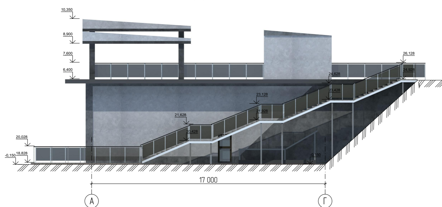
Фасад в осях А-Г
