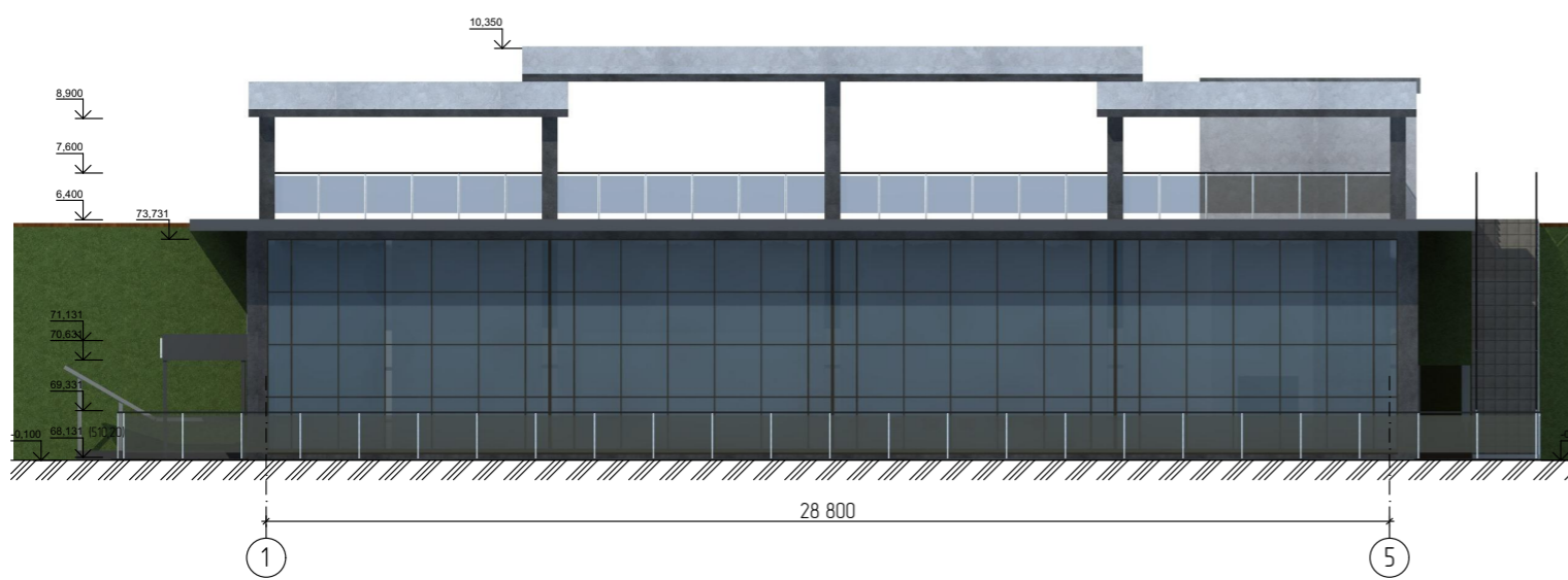
Фасад в осях 1-5
